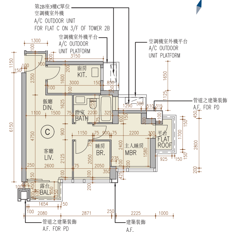
第2B座 3樓 C單位之樓面平面圖
